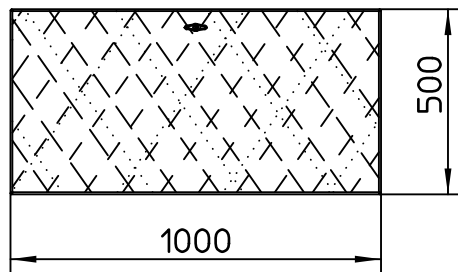
AllgSicht Maßstab 1:20
