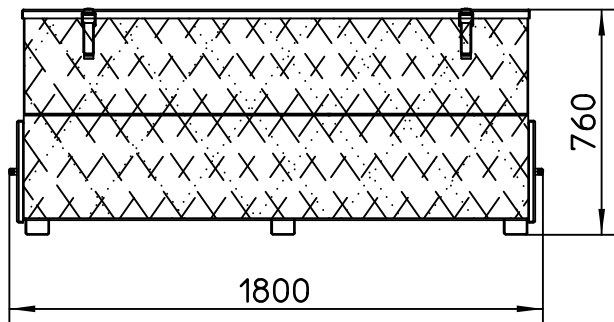
AllgSicht Maßstab 1:25
