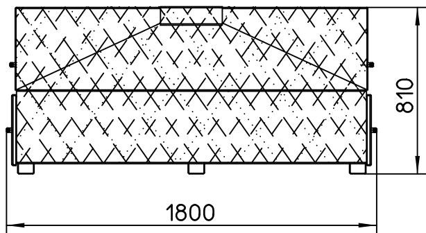
AllgSicht Maßstab 1:25
