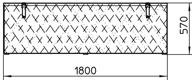
AllgSicht Maßstab 1:25
